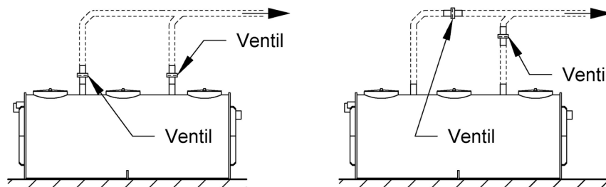
Figur PM/4. Alternativa ventilplaceringar, tömning - Typutförande
