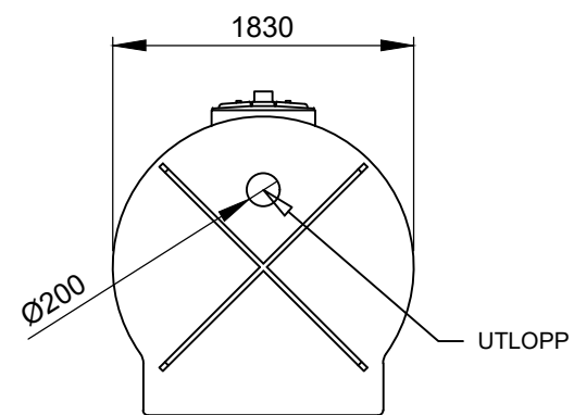
VY B-B
